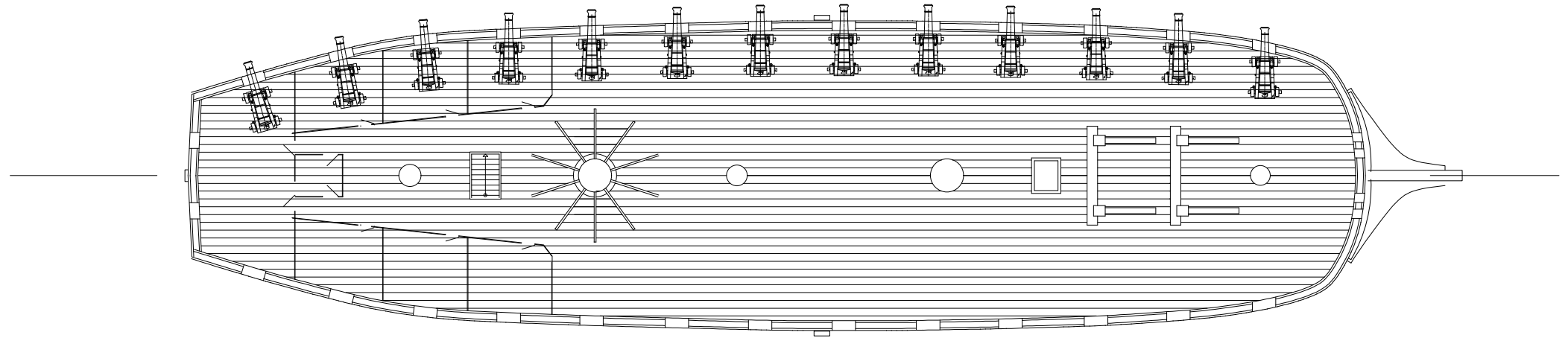
DANNEBROGE 1692-1710 DANSK ORLOGSSKIB BYGNING NR. 1 PÅ HOLMEN KONSTRUKTØR HENRIK SPANN OPTEGNING EJGIL THØSTESSEN
