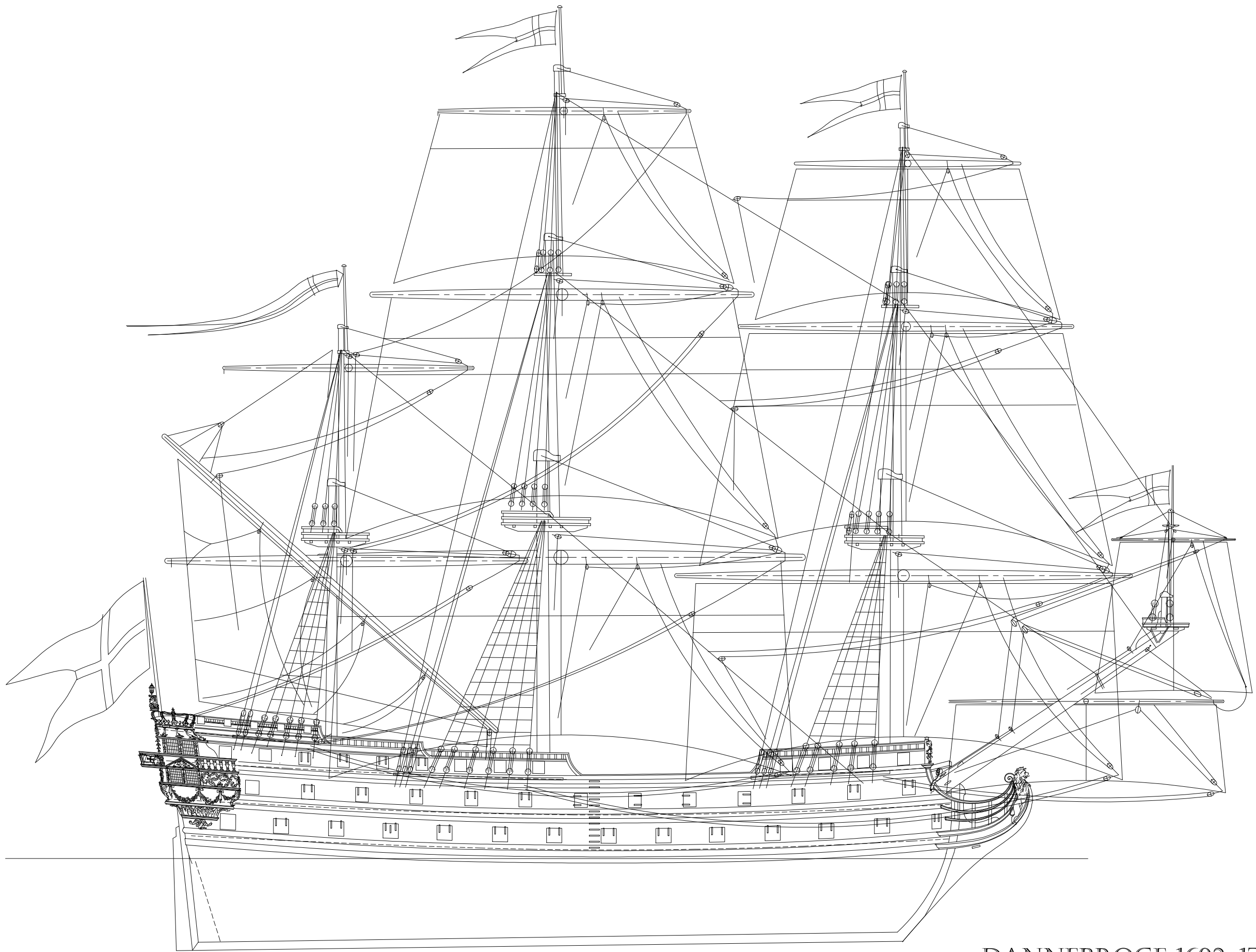
DANNEBROGE 1692-1710 DANSK ORLOGSSKIB BYGNING NR. 1 PÅ HOLMEN KONSTRUKTØR HENRIK SPANN OPTEGNING EJGIL THØSTESSEN
